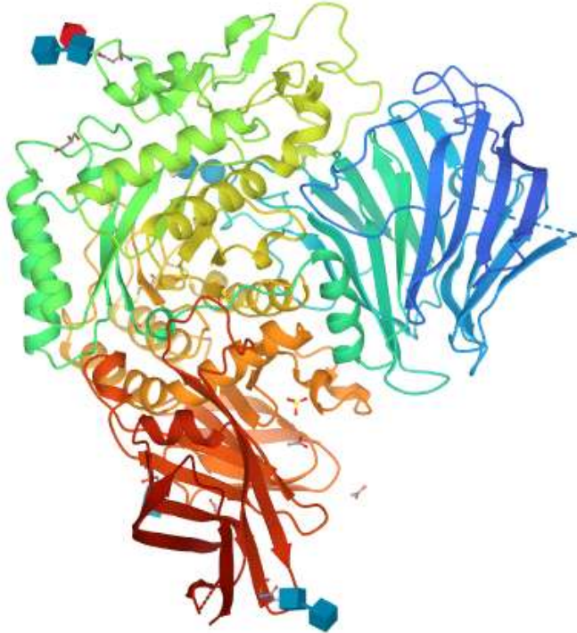
Lampiran 1. Struktur 3D Makromolekul \alpha -glukosidase dengan Kode PDB 3W37
