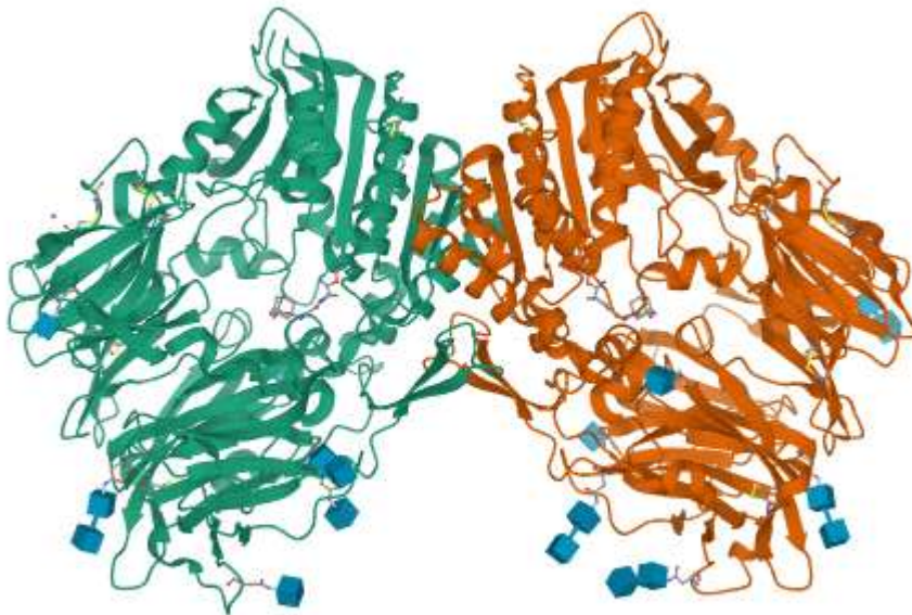
Lampiran 2. Struktur 3D Makromolekul DPP4 dengan Kode PDB 6B1E
