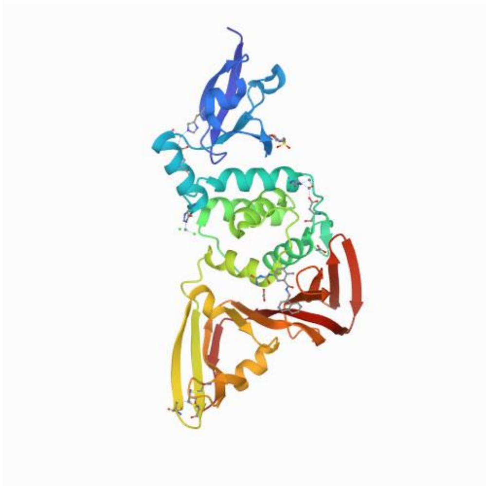
Struktur Makromolekul PLpro (PDB ID : 7JIT)
