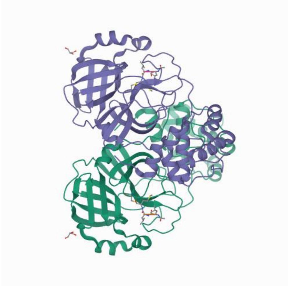
Struktur Makromolekul 3CLpro (PDB ID : 6XA4)
