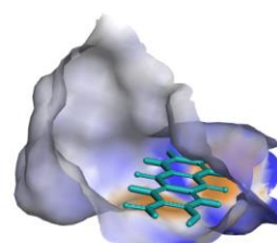
Nordamnacanthal
