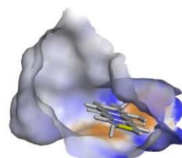
Soranjidiol
