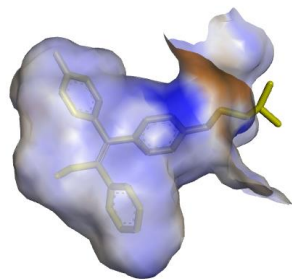
Native ligand 3ERT
