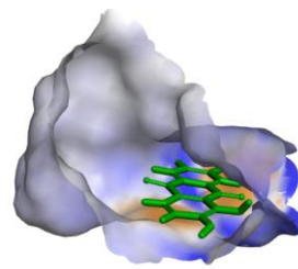
Alizarin
