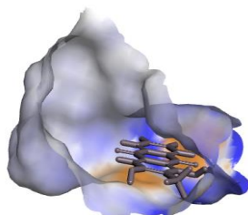
Rubiadin
