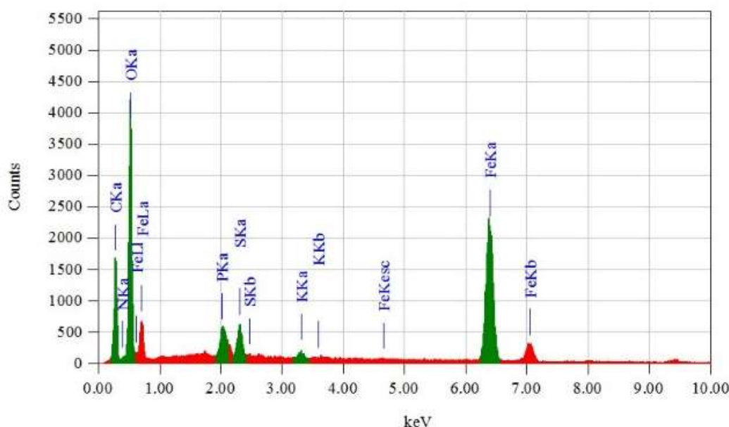
Gambar 4 Spektrum EDS nanopartikel besi
